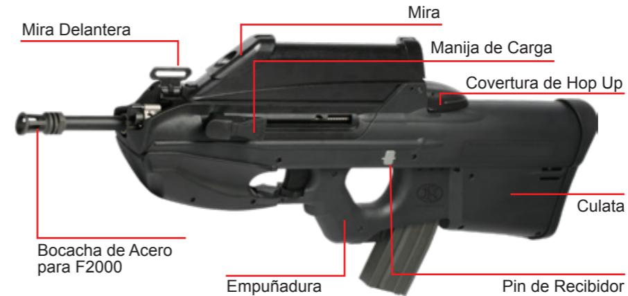
FN F2000 (Negro) FN F2000 FDE (Desierto)
